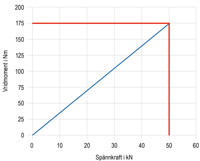
Åtdragningsmoment / spännkraft ESG 5 – 160 mm
