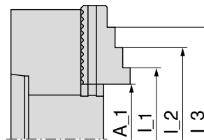
Hårda stegblocksbackar Stål 16MnCr5, sätthärdat
