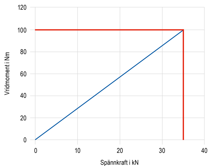
Åtdragningsmoment / spännkraft ESG 5 – 125 mm
