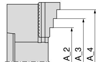
Hårda stegblocksbackar Stål 16MnCr5, sätthärdat
