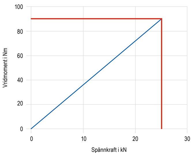
Åtdragningsmoment / spännkraft ESG 5 – 80 mm
