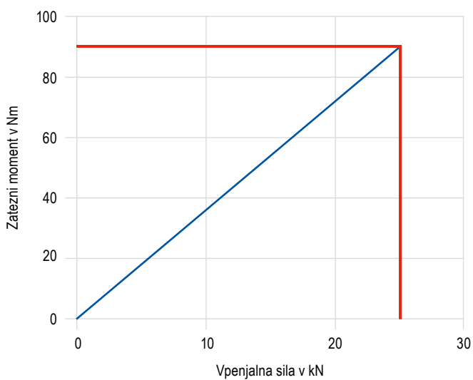
Zatezni moment / vpenjalna sila ESG 5 – 80 mm
