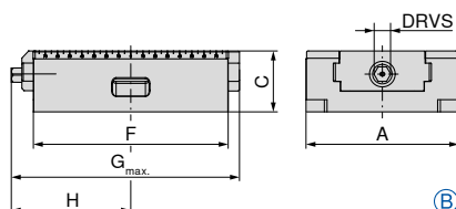
Zunanje aktivacijsko vreteno
