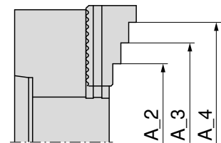
Trde stopničaste blokirne čeljusti jeklo 16MnCr5, kaljene
