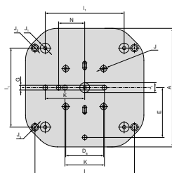
Trikotni vpenjalni stolp
