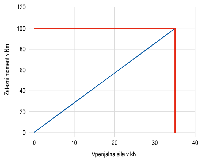
Zatezni moment / vpenjalna sila ESG 5 – 125 mm
