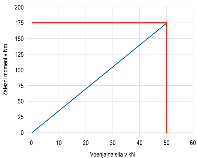
Zatezni moment / vpenjalna sila ESG 5 – 160 mm
