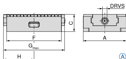
Notranje aktivacijsko vreteno
