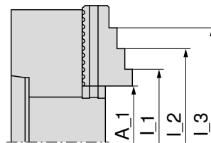
Tvrdé stupňovité blokové čeluste ocel 16MnCr5, cementovaná, kalená
