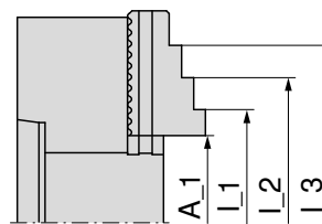
Getrapte harde bekken Staal 16MnCr5, oppervlakte gehard
