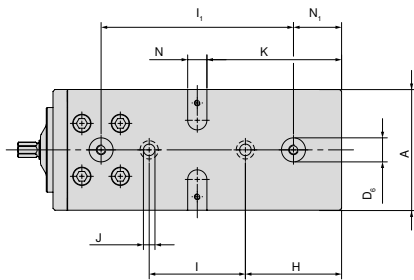
Basisbreedte 125 mm en lengte 300 mm
