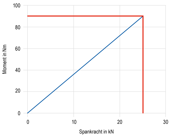
Aantrekmoment / spankracht ESG 5 – 80 mm
