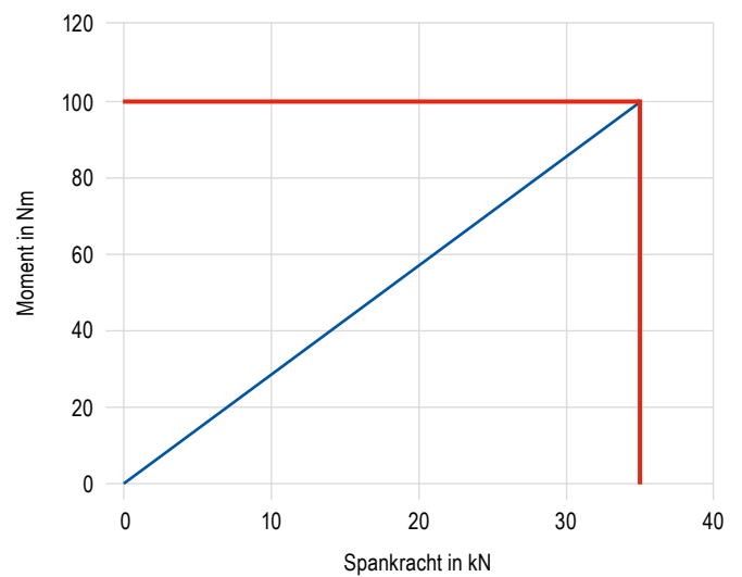
Aantrekmoment / spankracht ESG 5 – 125 mm
