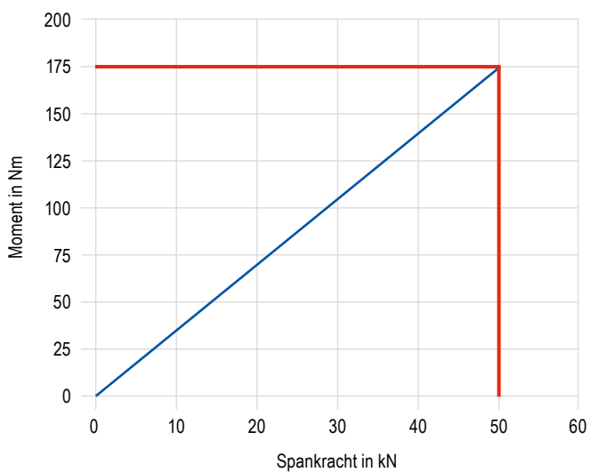
Aantrekmoment / spankracht ESG 5 – 160 mm
