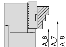
Stellen van de grondbekken 2
