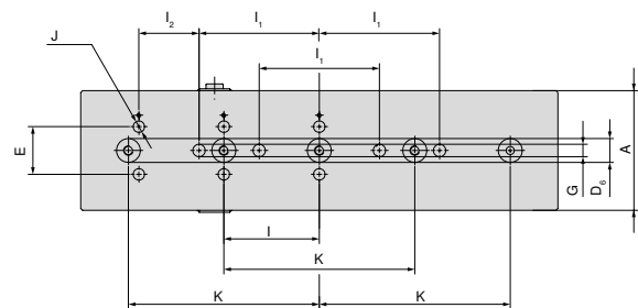
Basisbreedte 125 mm en lengte 500 mm
