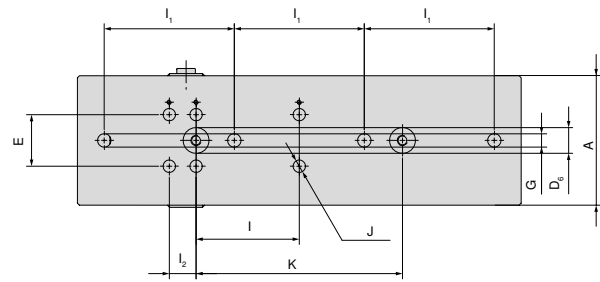
Basisbreedte 125 mm en lengte 430 mm
