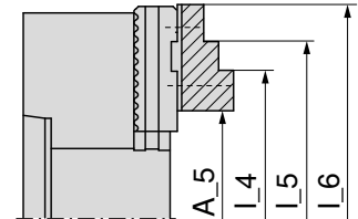
Stellen van de grondbekken 1
