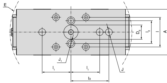
Basisbreedte 80 mm en lengte 190 mm
