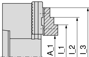
Stellen van de grondbekken 2
