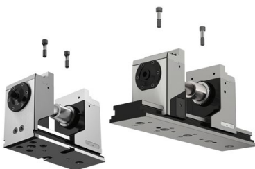
Opspannen met twee pasbouten Ø 12 17 / M12 Artikel-nr. 80 895 019
