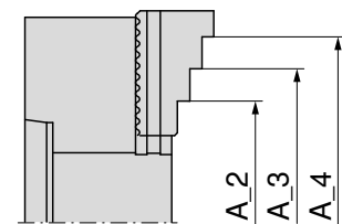
Getrapte harde bekken Staal 16MnCr5, oppervlakte gehard
