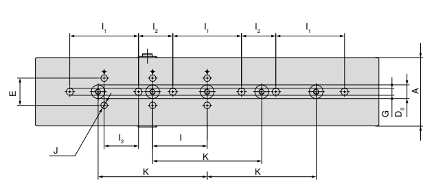
Basisbreedte 125 mm en lengte 630 mm
