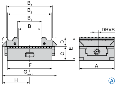
Indvendig betjeningsspindel
