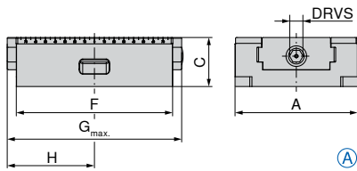
Indvendig betjeningspindel
