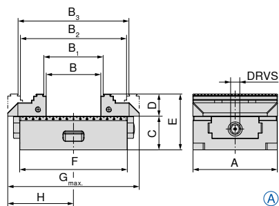
Вътрешен задвижващ шпиндел
