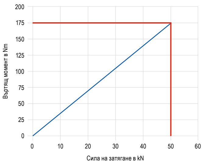
Затягащ момент/сила на затягане ESG 5 – 160 мм
