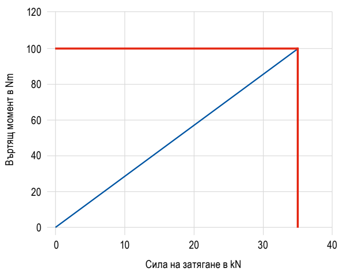
Затягащ момент/сила на затягане ESG 5 – 125 мм
