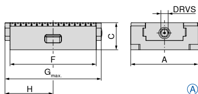
Вътрешен задвижващ шпиндел
