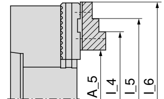
Основна позиция на челюстите 1
