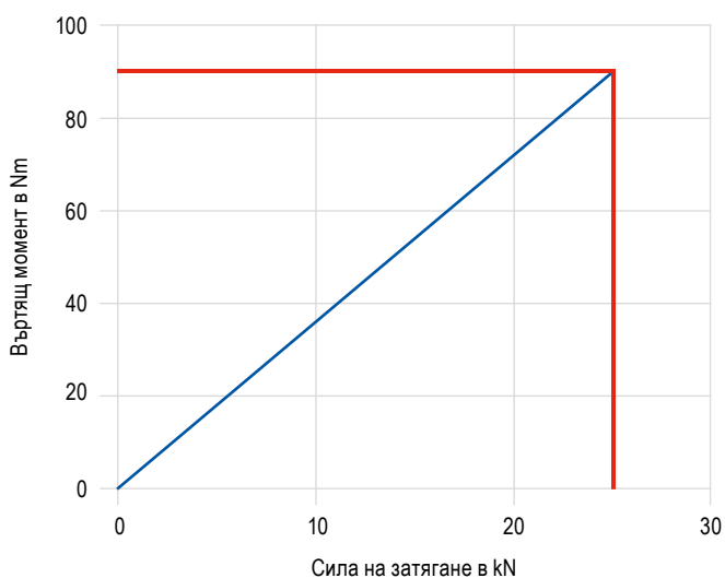
Затягащ момент/сила на затягане ESG 5 – 80 мм
