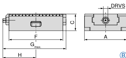
Външен задвижващ шпиндел
