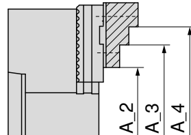
Основна позиция на челюстите 1
