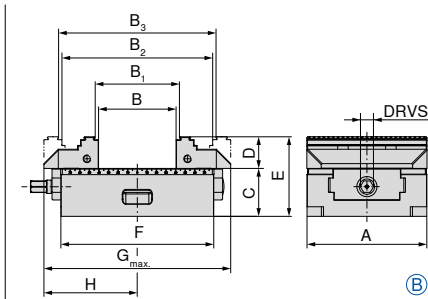
Външен задвижващ шпиндел
