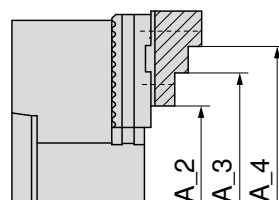
Posição do mordente base 1
