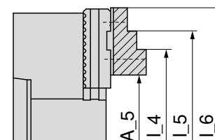
Posição do mordente base 1
