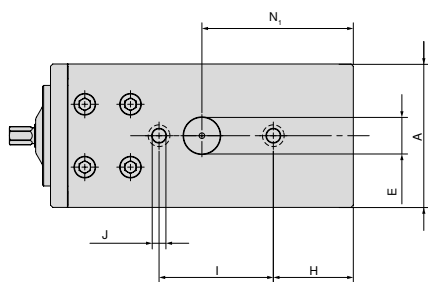
Base largura 125 mm e comprimento 265 mm
