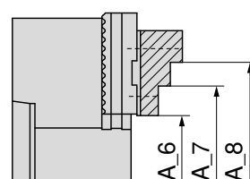
Posição do mordente base 2
