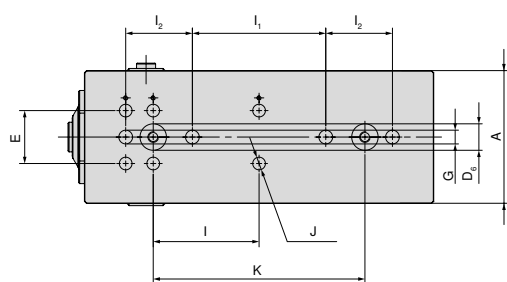
Base largura 125 mm e comprimento 330 mm
