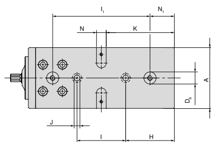
Base largura 125 mm e comprimento 300 mm
