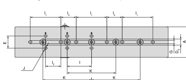
Base largura 125 mm e comprimento 630 mm
