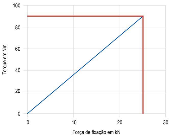
Torque de aperto / Força de fixação ESG 5 – 80 mm
