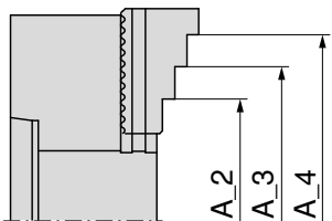
Mordentes escalonados duros Aço 16MnCr5, cementado
