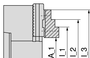
Posição do mordente base 2
