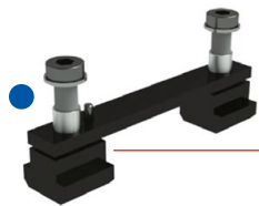
Hizalama ve merkezleme seti mesafesi 100 mm
