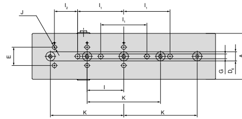
Taban genişliği 125 mm ve uzunluk 500 mm
