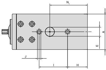
Taban genişliği 125 mm ve uzunluk 265 mm
