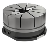
Pinza in alluminio con il profilo del pezzo integrato nella MNG tonda
