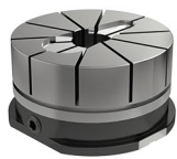
Alu-spændetang med indarbejdet emneform til MNG rund
