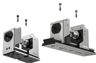
Opspænding med to passkruer Ø 12 17 / M12
