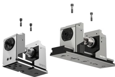
Aufspannen mit zwei Passschrauben Ø 12 17 / M12 Artikel-Nr. 80 895 019
