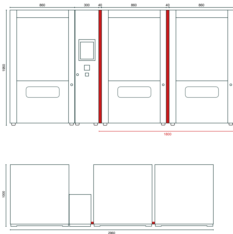
Tool-O-Mat 80 – Hoofd unit + Uitbreidings unit + Uitbreidings unit
