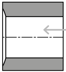
Hinterdrehen Differentialgehäuse
