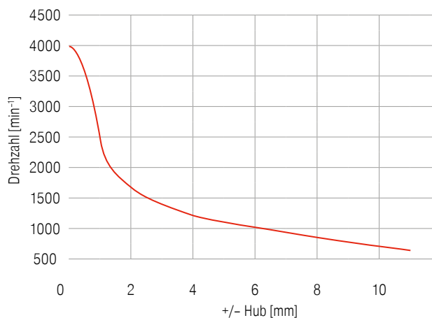
Max. Hub-Drehzahldiagramm bis 1 kg Aufsatzwerkzeug inkl. Adapter
