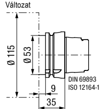
UAS-115-HSK-A63-...-L35
