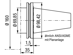
UAS-160-CAT-FC50-...-L35 Variante
