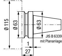
UAS-115-BT-FC40-...-L27 Variante
