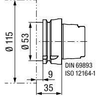
UAS-115-HSK-A63-...-L35 Variante
