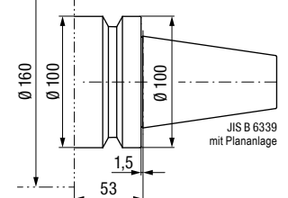
UAS-160-BT-FC50-...-L53 Variante
