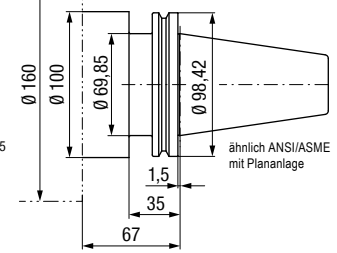
UAS-160-CAT-FC50-...-L67 Variante
