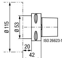
UAS-115-PSC63-...-L42 Variante
