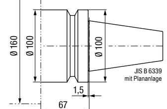
UAS-160-BT-FC50-...-L67 Variante
