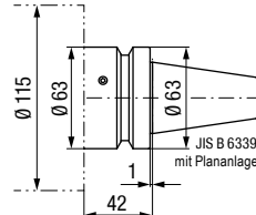
UAS-115-BT-FC40-...-L42 Variante
