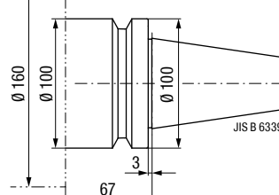
UAS-160-BT50-...-L67 Variante
