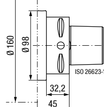
UAS-160-PSC80-...-L45 Variante
