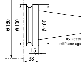
UAS-160-BT-FC50-...-L38 Variante
