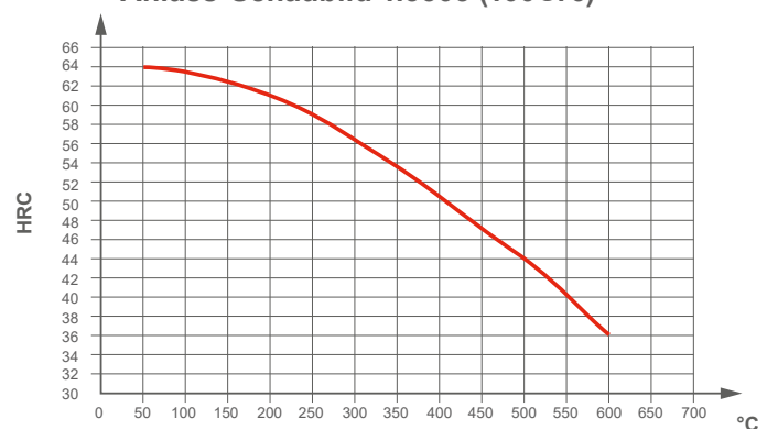
Anlass-Schaubild 1.3505 (100Cr6)
